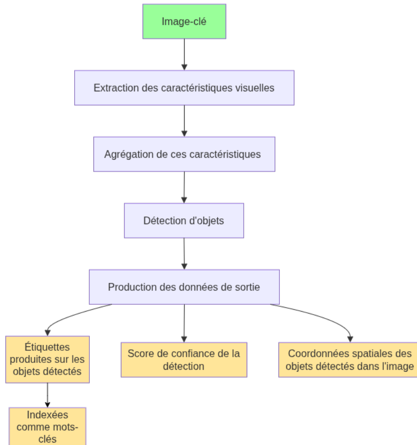
FIG. 3 : Processus de détection d'objets de YOLO
