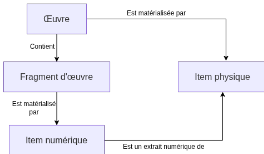
FIG. 4 : Intégration du Fragment au modèle de données
